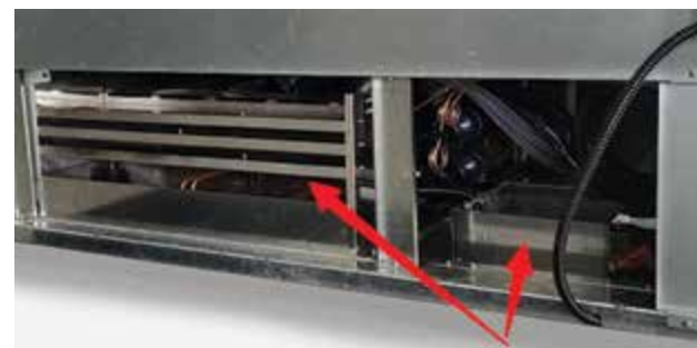
Élément chauffant du bac de récupération pour l'évaporation de la condensation
